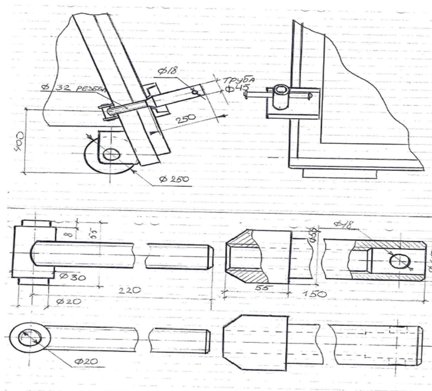
Joonis 3. Tellija nõuded uuele tagaluugi kinnituse lahendile.
