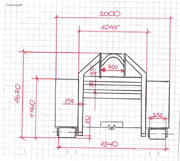
Joonis 2. Tellija nõuded konteineri mõõtudele (eestvaade)
