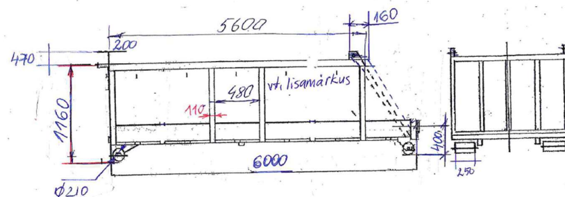
Joonis 1. Tellija nõuded konteineri mõõtudele (küljvaade, vaade tagant)
