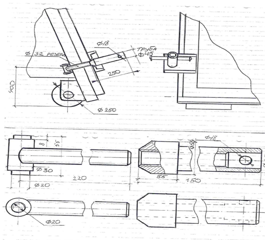
Joonis 3. Tellija nõuded uuele tagaluugi kinnituse lahendile.
